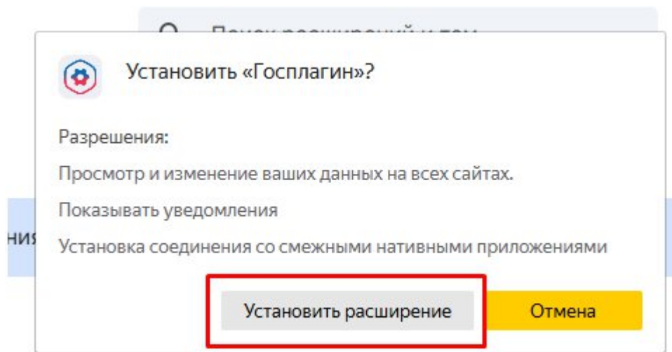
Рисунок 15 – Установка «Госплагина»
