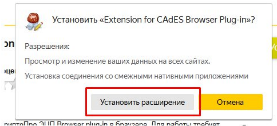
Рисунок 13 – Установить расширение
